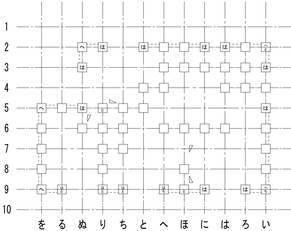
2階柱壁伏図
