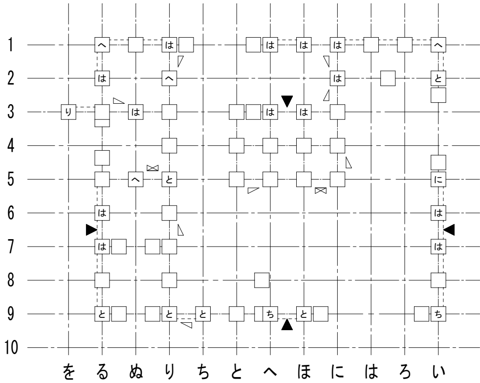
1階柱壁伏図
